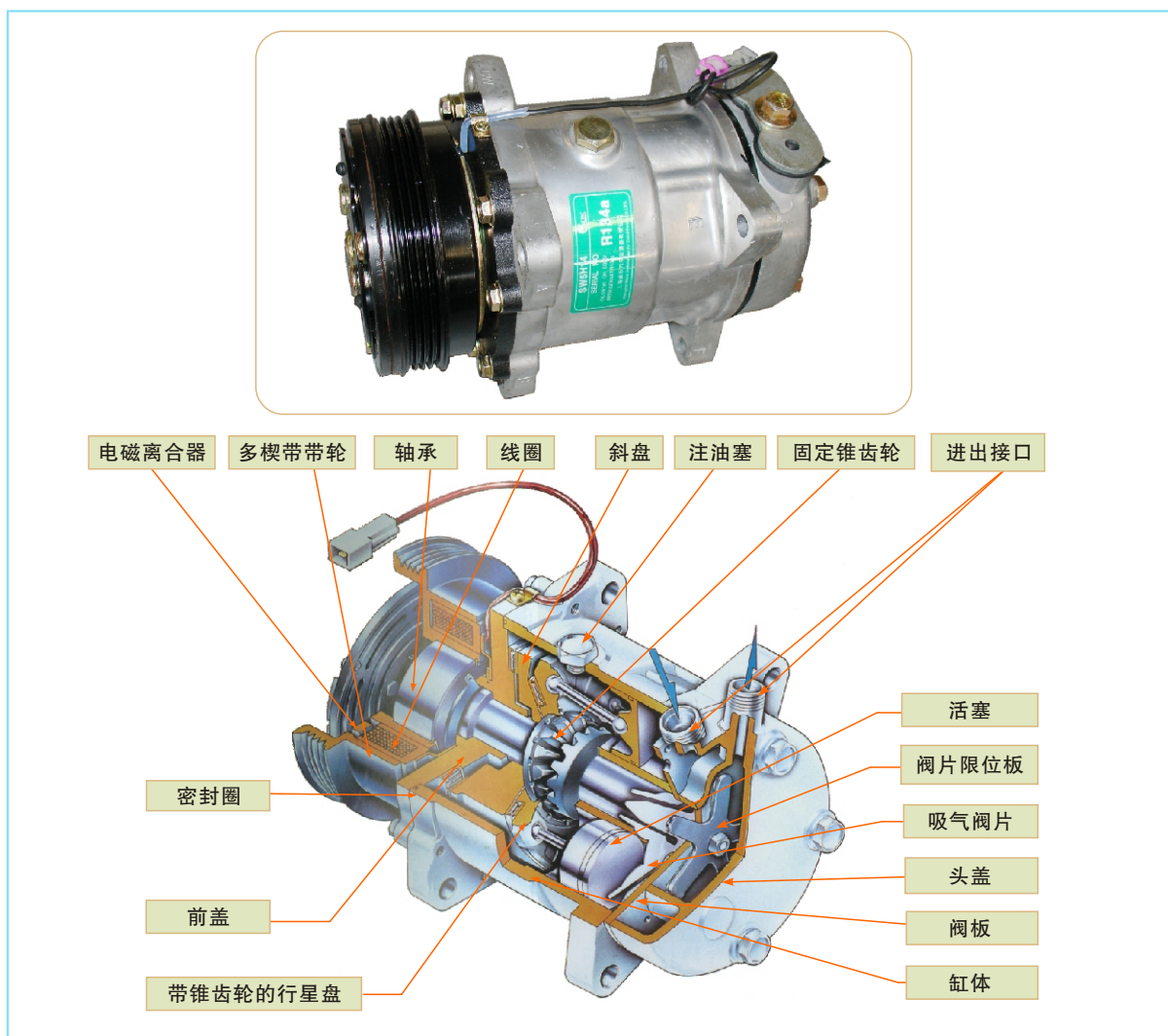
图8-2 摇板式活塞压缩机
