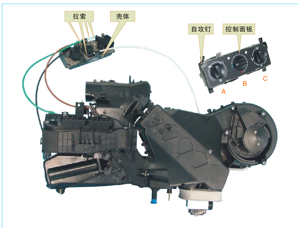
图8-12 空调控制装置的分解图
