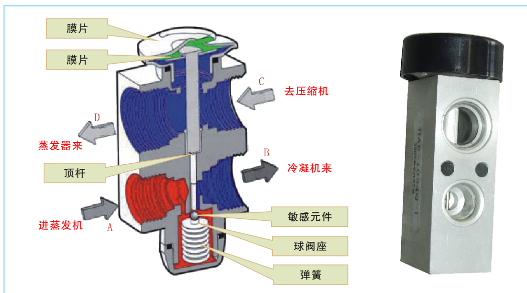
图8-8 膨胀阀
