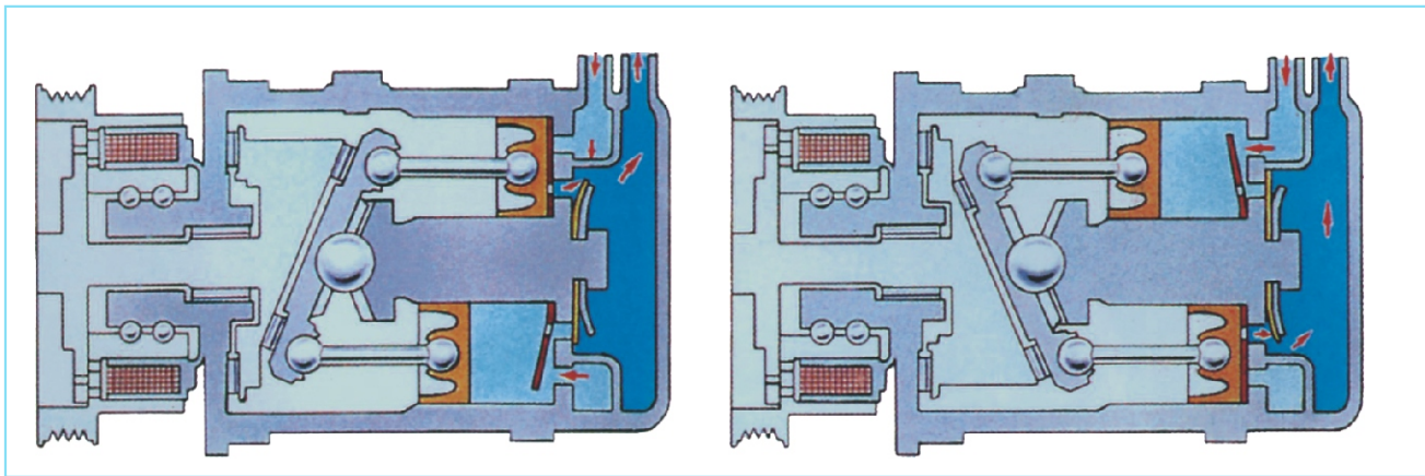
图8-3 压缩机工作过程
