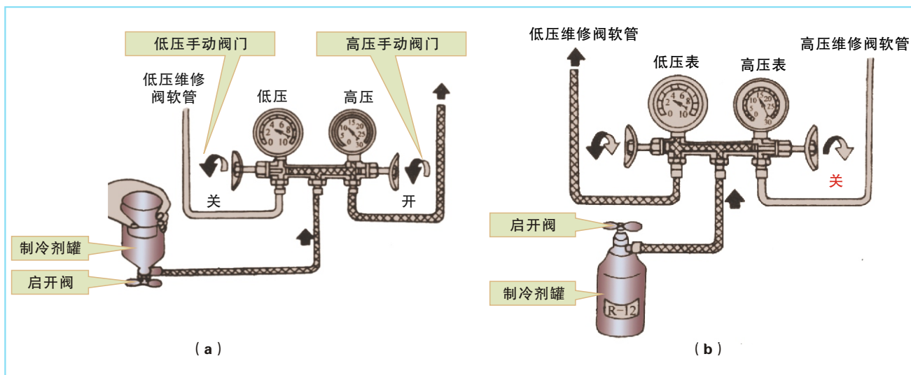
图8-17 制冷剂的充注
