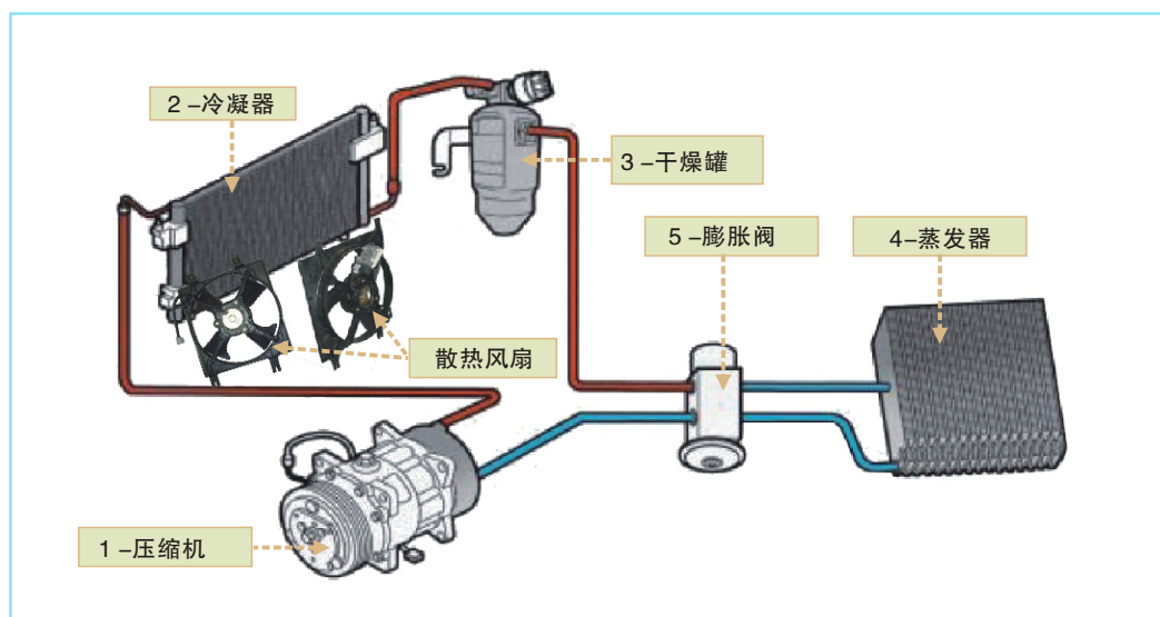
图8-1 制冷系统工作原理
