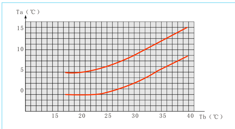
图8-13 温度曲线图
