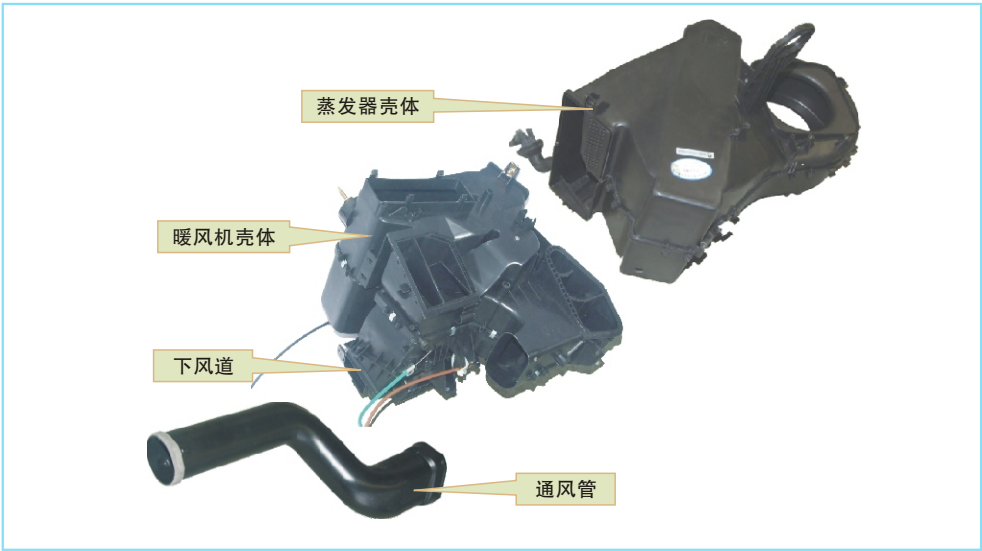
图8-10 暖风机组的分解图
