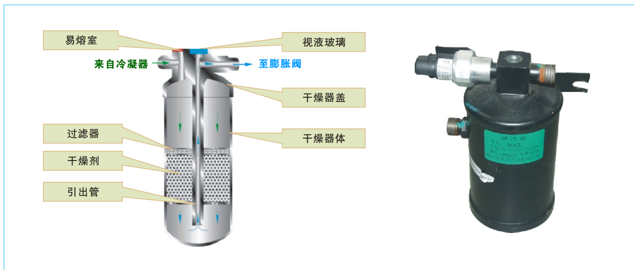
图8-9 储液干燥罐结构与实物图
